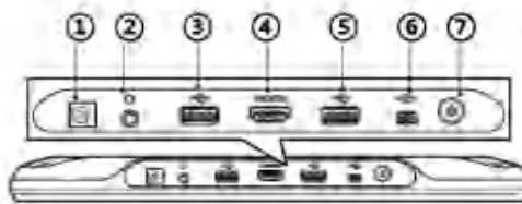
Figure 2-3 D1 Pro Tablet, Top View
